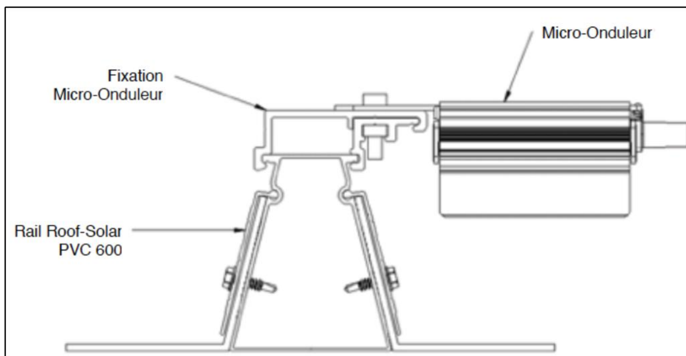
Figure 27 – Micro-onduleur
