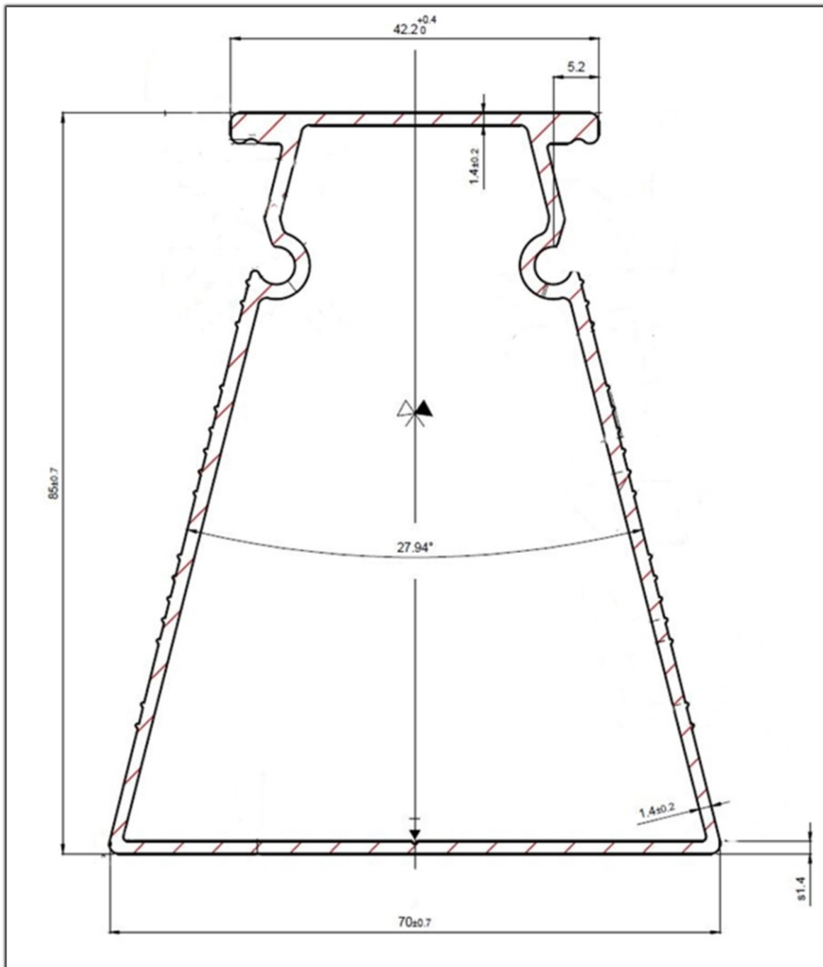
Figure 6 – Profil trapézoïdal
