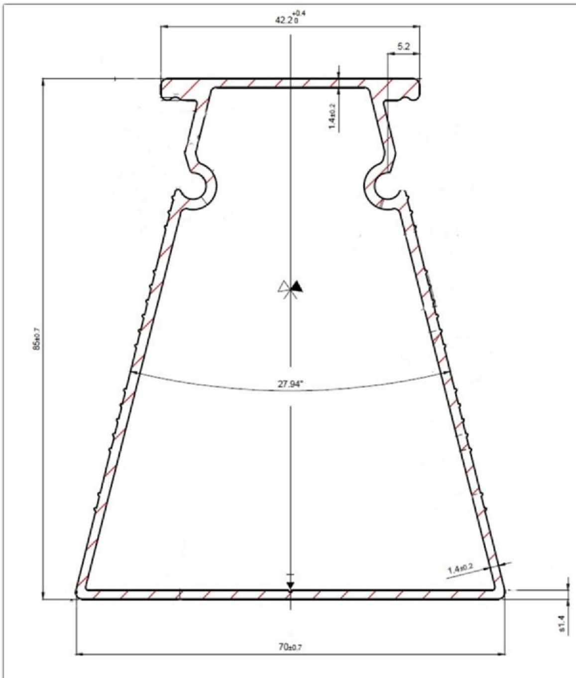
Figure 4 – Profil trapézoïdal
