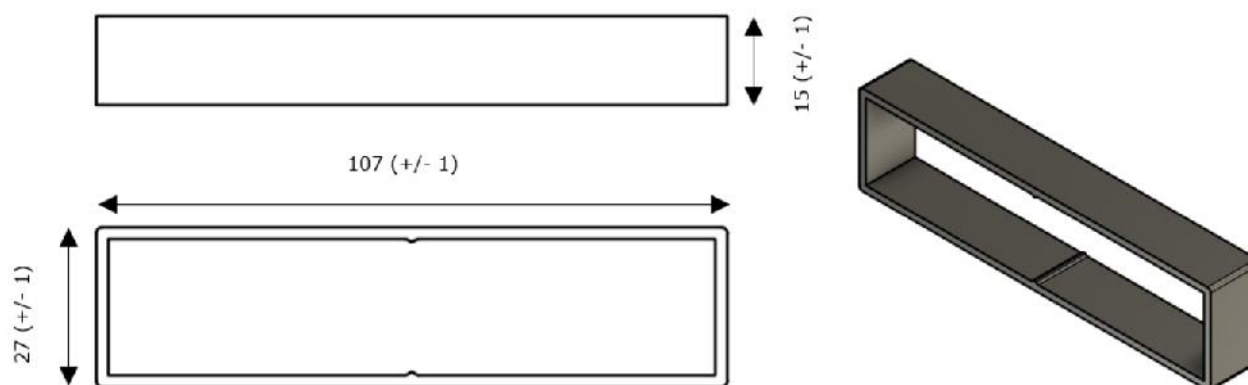
Figure 18 - Cale rotule du kit d'inclinaison du procédé ROOF-SOLAR BITUME TAN GP – Plat & Incliné
