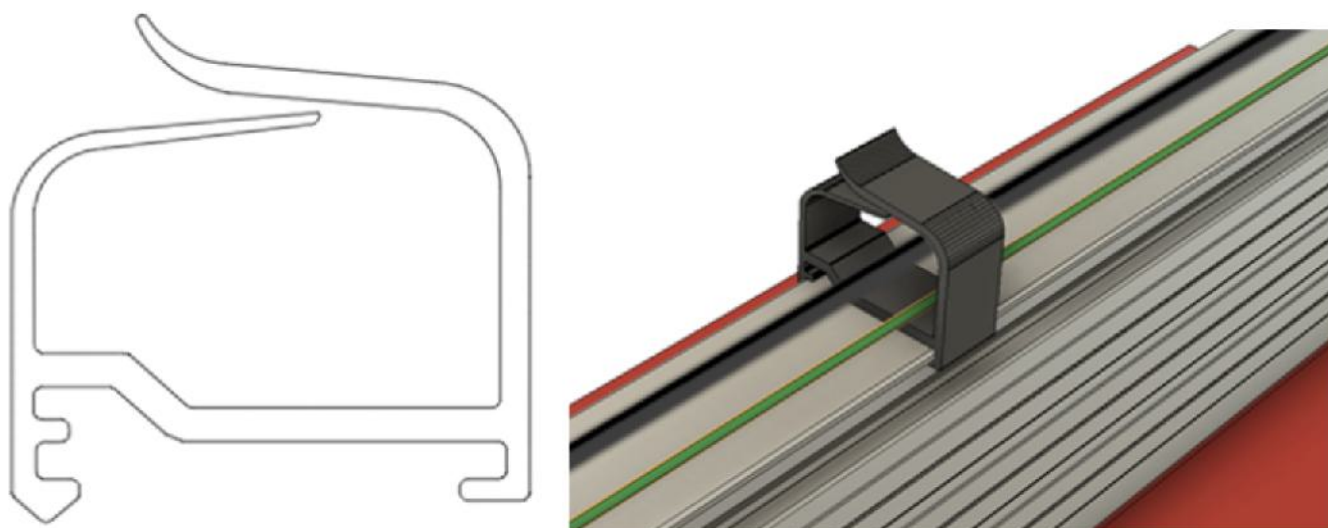
Figure 12 - Collier Passe Câbles du procédé ROOF-SOLAR BITUME TAN GP – Plat & Incliné
