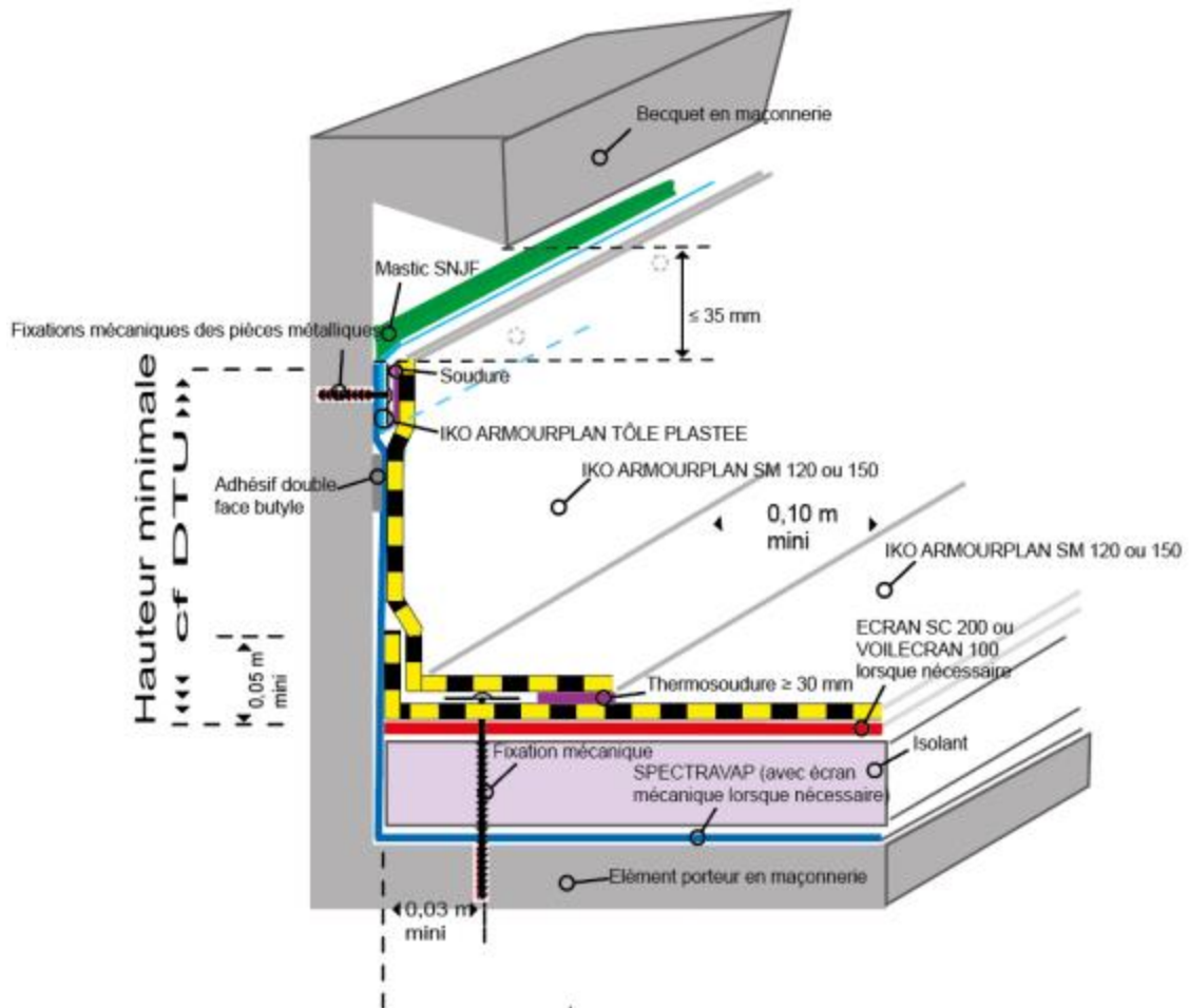
Figure 27 - Relevés d'étanchéité <math>< 500\text{ mm}</math> avec pare-vapeur polyéthylène SPECTRAVAP
