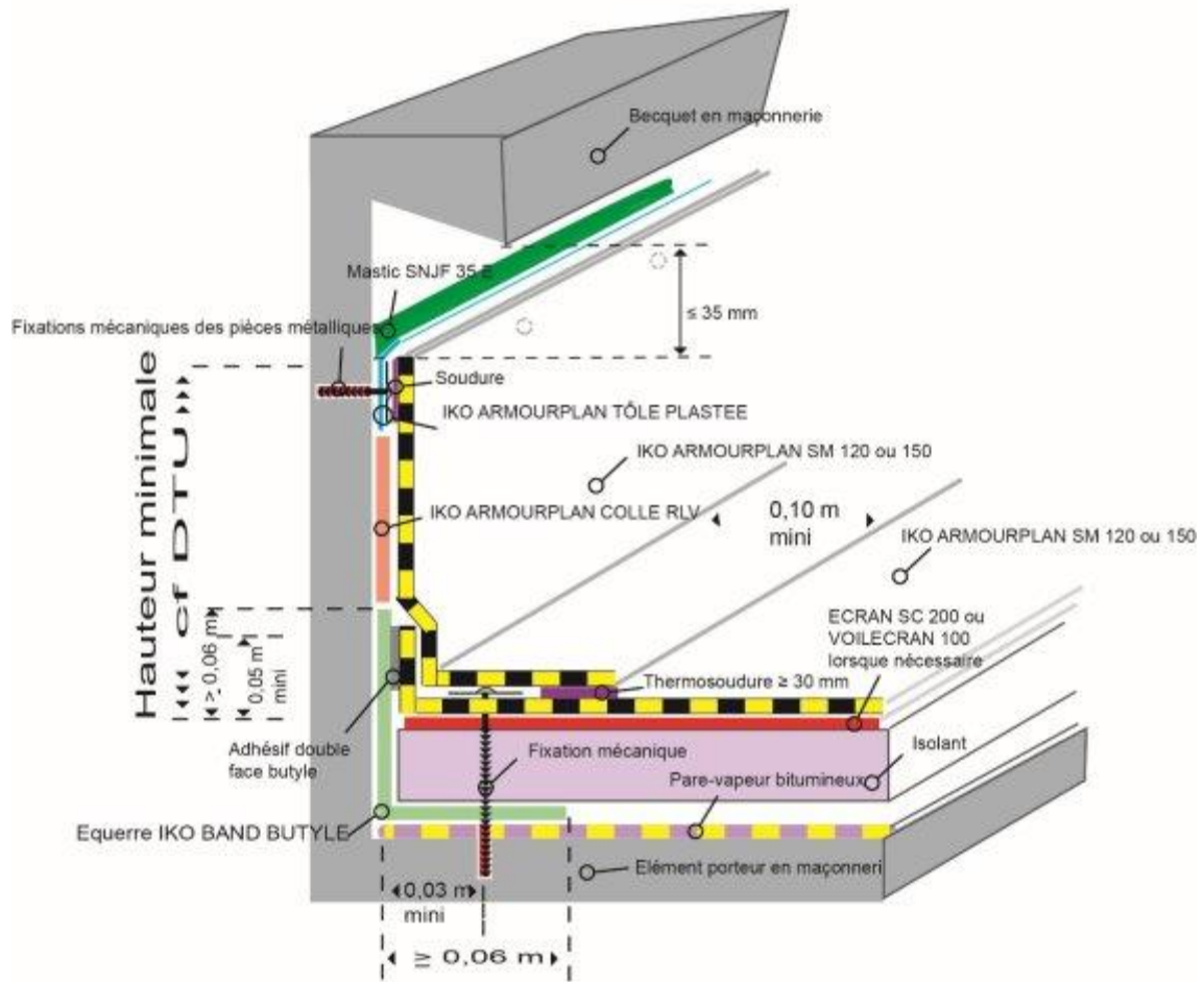
Figure 13 – Relevé d'étanchéité avec tôle plastée (maçonnerie avec isolation)
