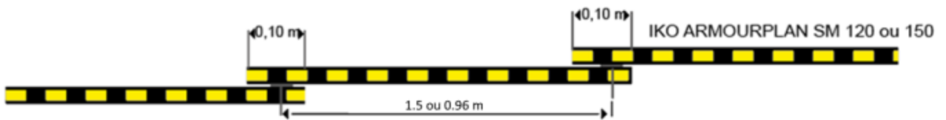
Figure 1 – Principe de fixation mécanique en lisière
