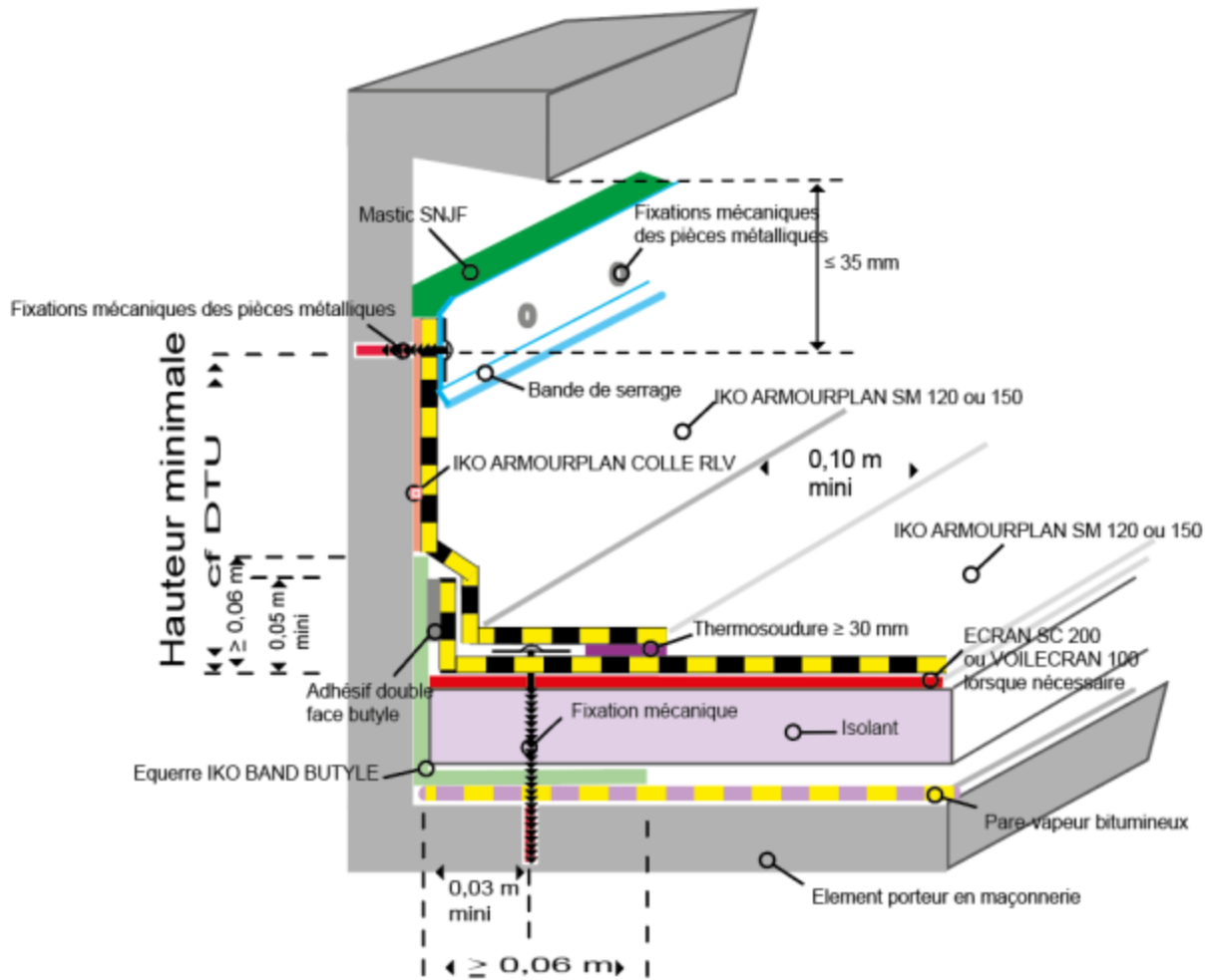
Figure 14 - Relevés d'étanchéité avec bande de serrage (maçonnerie)
