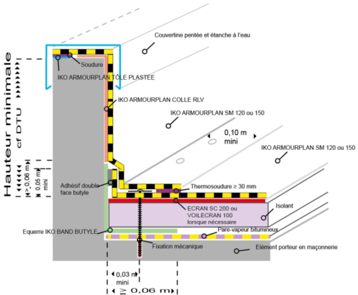
Figure 16 – Relevés d'étanchéité sous couvertine sur support en maçonnerie NB : les cotes des relevés doivent être conformes à celles du Fascicule du CSTB 3502
