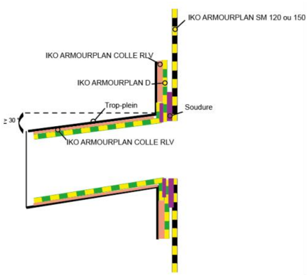
Figure 21 - Habillage des trop-pleins
