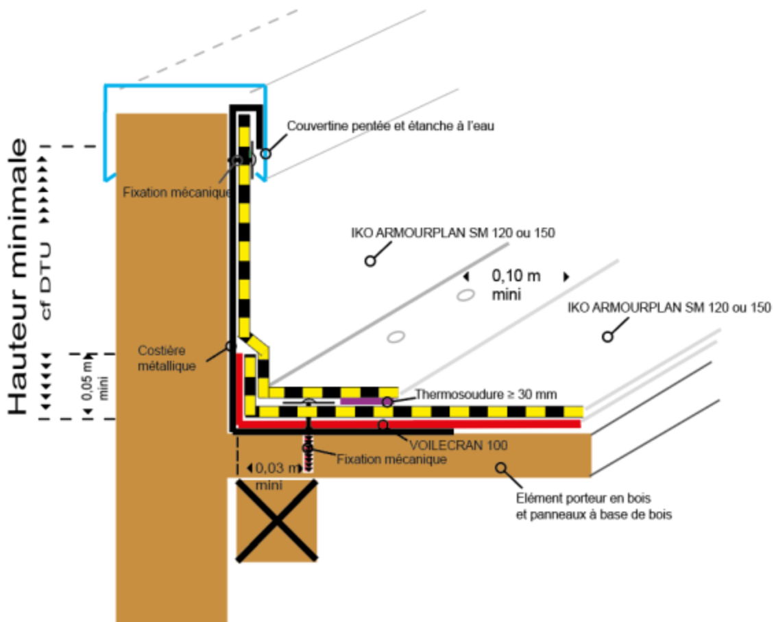
Figure 26 – Relevés d'étanchéité sous couvertine (bois et panneaux à base de bois) NB : les cotes des relevés doivent être conformes à celles du Cahier du CSTB 3502
