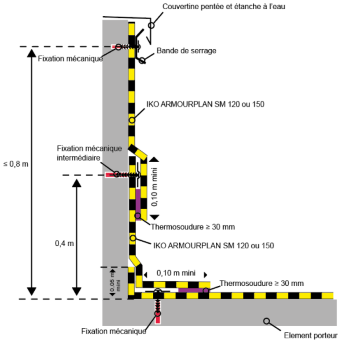
Figure 31 - Relevés d'étanchéité de grande hauteur > 50 cm et ≤ 80 cm avec lignes de fixations intermédiaires
