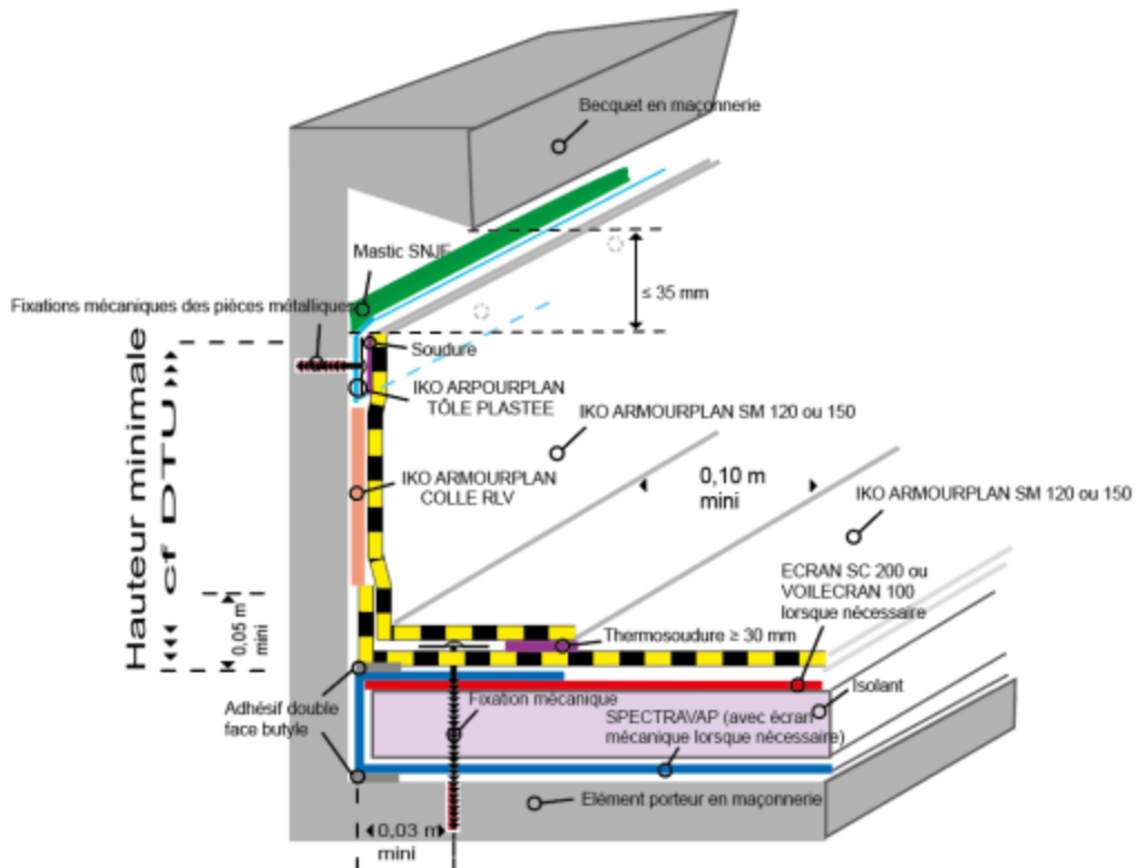
Figure 27 - Relevés d'étanchéité <math>< 500\text{ mm}</math> avec pare-vapeur polyéthylène SPECTRAVAP
