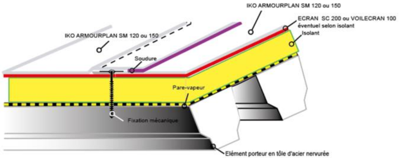
Figure 8 – Fixation mécanique en lisière de partie courante
