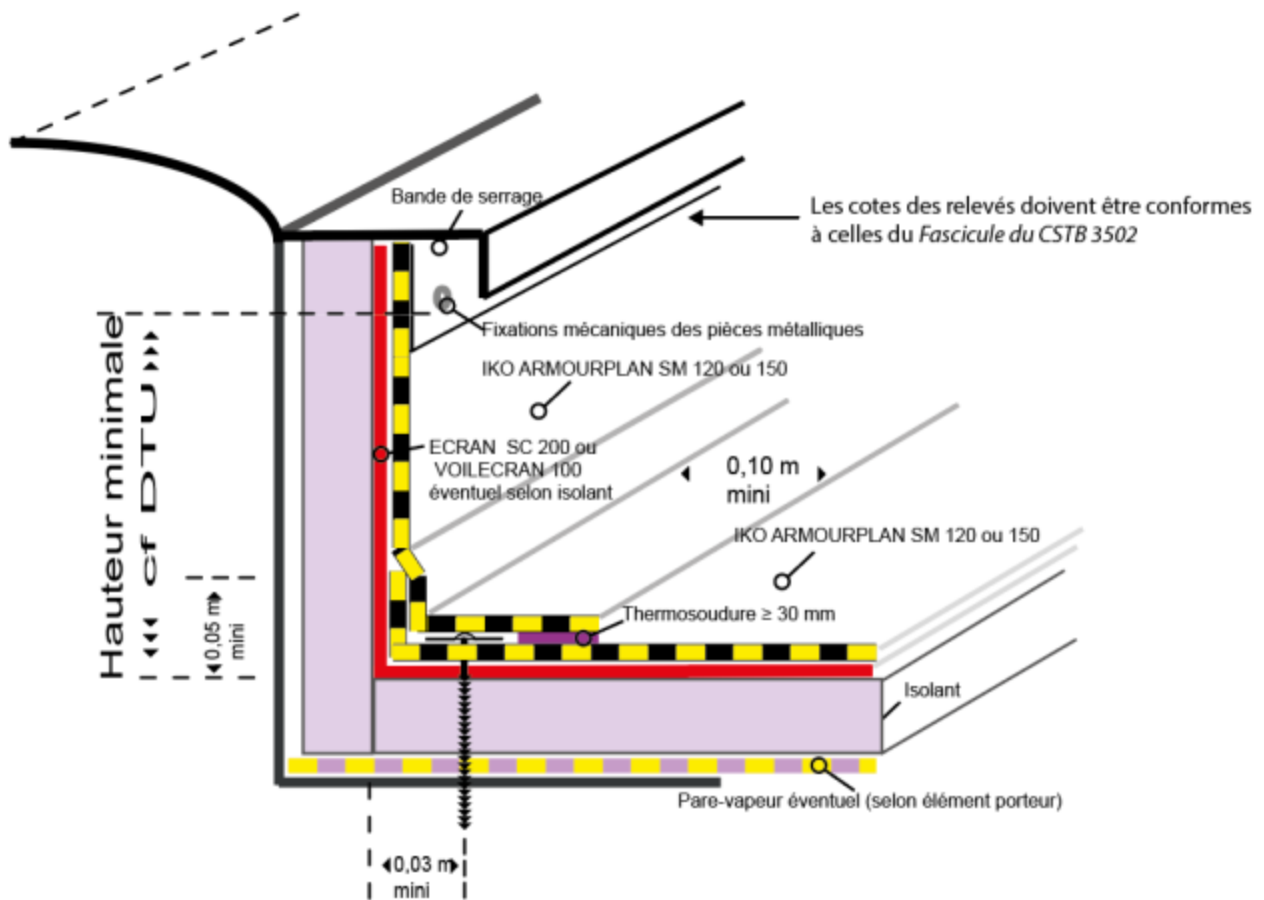
Figure 12 – Relevés d'étanchéité sur costière métallique de lanterneaux
