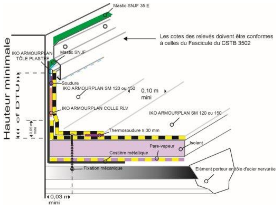
Figure 11 – Relevés d'étanchéité contre murs avec bande soline
