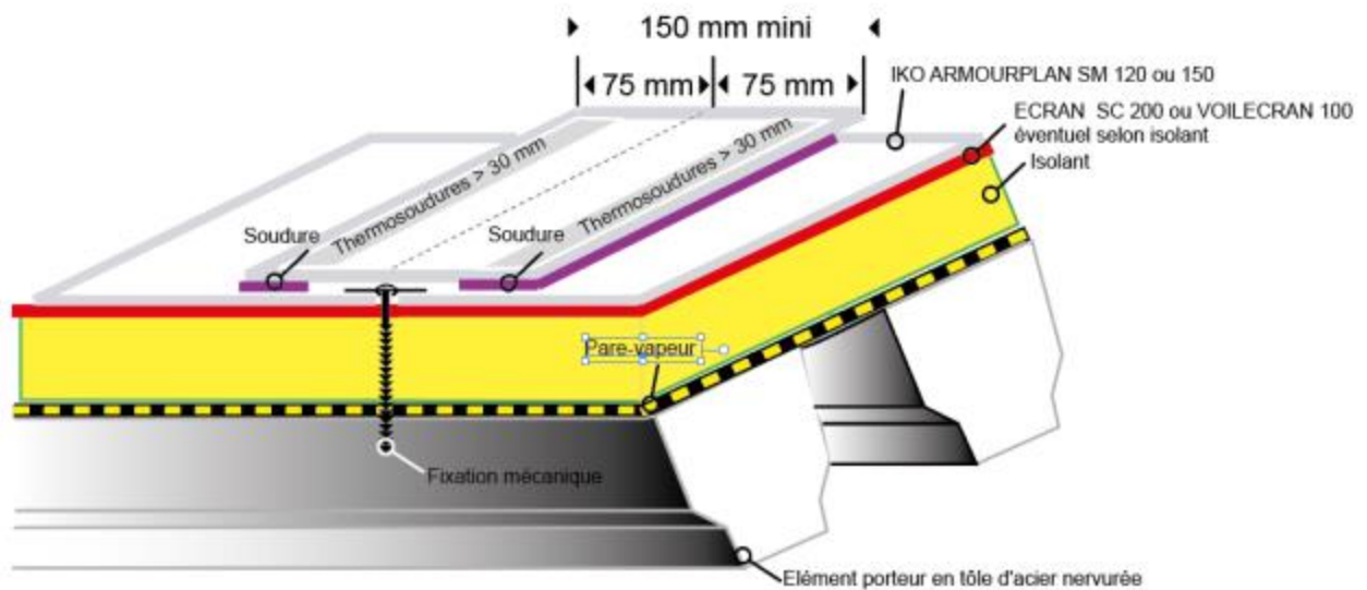
Figure 9 – Fixation mécanique avec bande de pontage en partie courante
