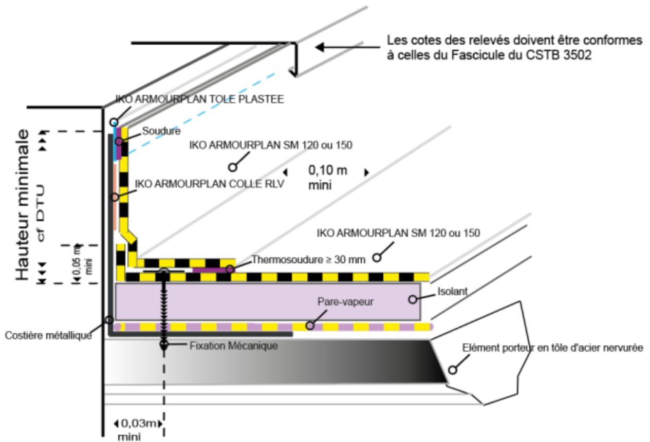
Figure 10 – Relevés d'étanchéité contre acrotères avec couvertine (TAN)
